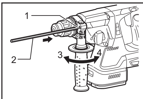
► 1. Orificio 2. Calibrador de profundidad 3. Aflojar 4. Apretar
