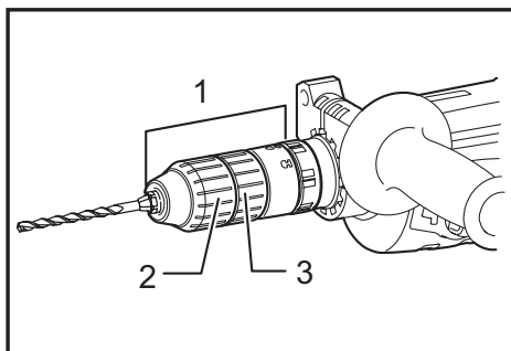
► 1. Mandril de cambio rápido 2. Base de mandril 3. Anillo
