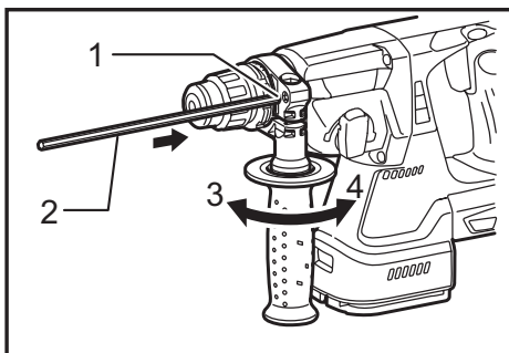
► 1. Orifice 2. Jauge de profondeur 3. Desserrer 4. Serrer
